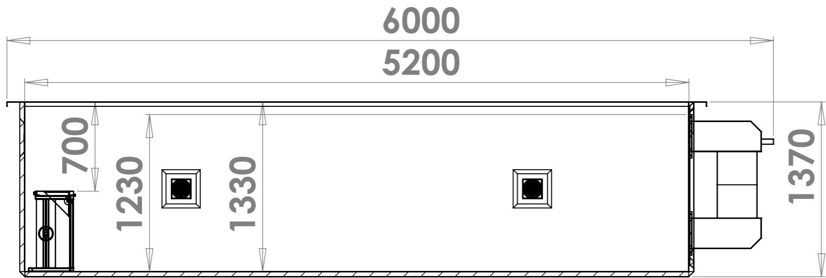
COUPE B-B
