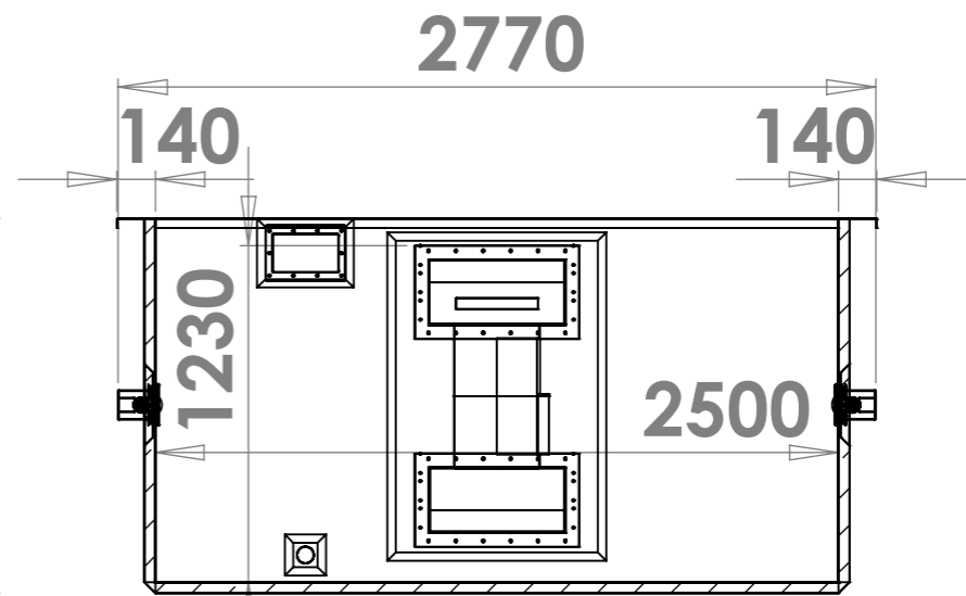
COUPE B-B
